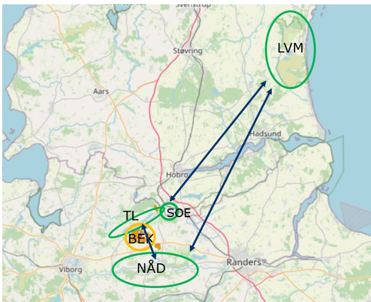
Figur 7-5 Beliggenhed af opholdssteder for Tjælgasædgås: LVM = Lille Vildmose, TL = Tjele Langsø, NÅD = Nørreådal, SOE = Sønder Onsild Enge, BEK = Udkast til Bekendtgørelses foreslåede udpegede areal. Pilene indikerer potentielle flyveruter mellem opholdssteder.
